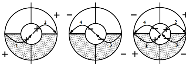
Рис. 3. Движение магнитных потоков Земли
