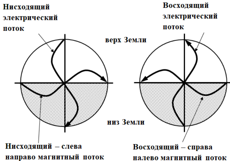
Рис. 1. Восходящие и нисходящие потоки электрических и магнитных сил
