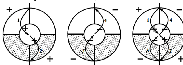
Рис. 2. Движение электрических потоков Земли
