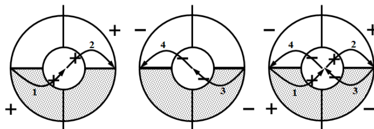
Рис. 3. Движение магнитных потоков Земли
