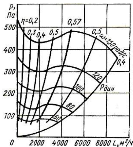
Рисунок 2 – Характеристика вентилятора при разных частотах вращения
