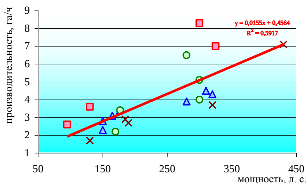
Рисунок 4 – Зависимость производительности агрегатов от мощности двигателя трактора
