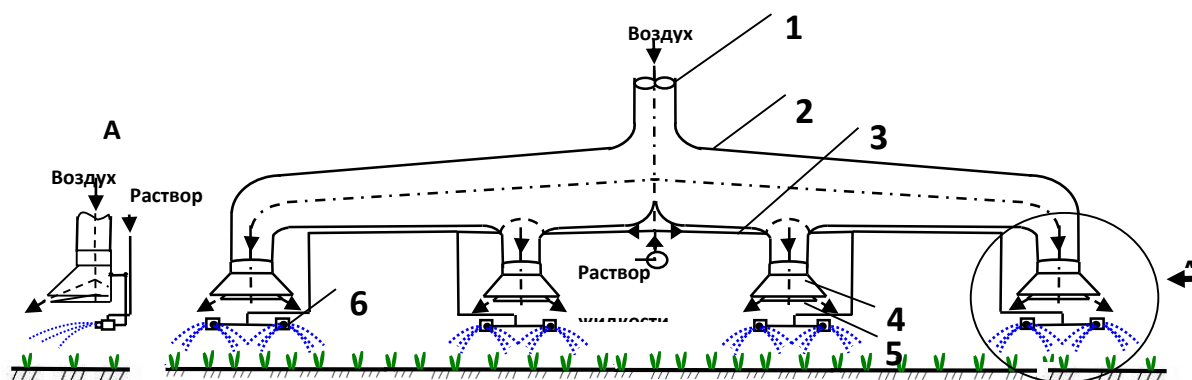
Рисунок 1 – Воздухораспределительная система штангового опрыскивания растений с пневмогидравлическими устройствами
