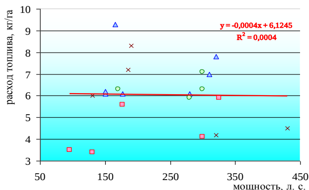
Рисунок 5 – Зависимость удельного расхода топлива от мощности двигателя трактора
