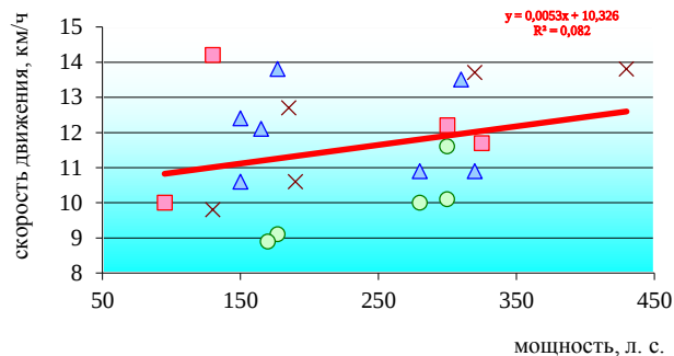
Рисунок 3. Зависимость рабочей скорости движения от мощности двигателя трактора
