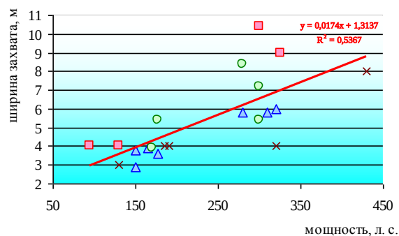
Рисунок 2. Зависимость ширины захвата агрегатов от мощности двигателя трактора
